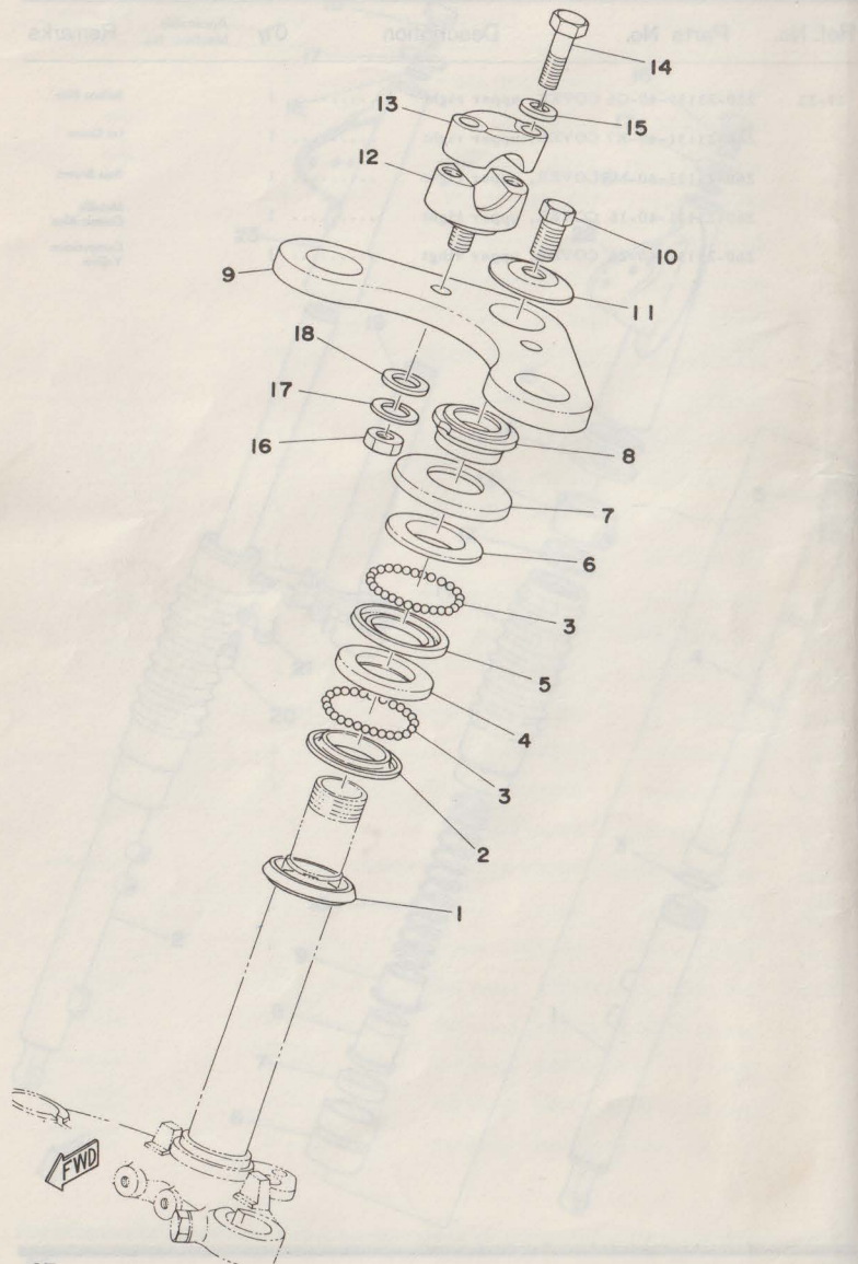
Fig. 18 STEERING
