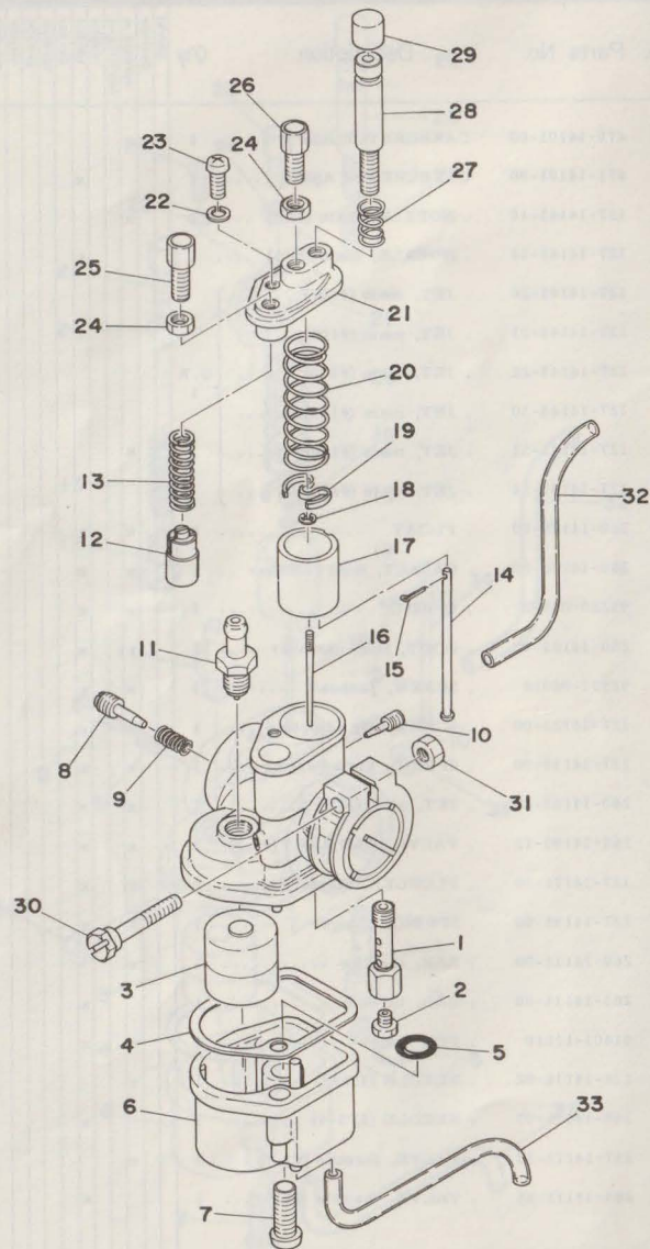
Fig. 10 CARBURETOR
