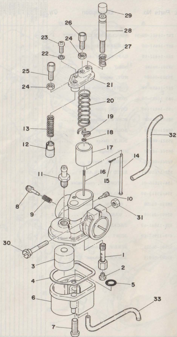
Fig. 10 CARBURETOR
